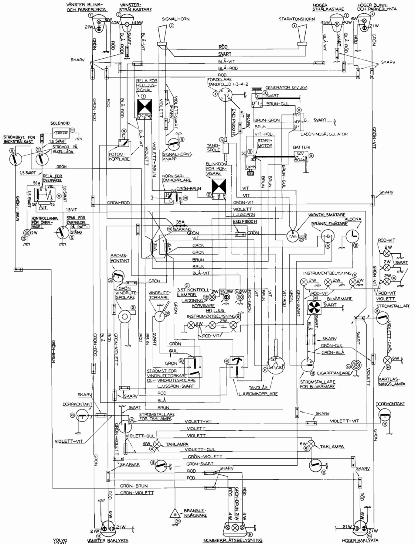
Bildtafel IV Elektrischer Schaltplan ab Fahrgestell-Nr. 12501
