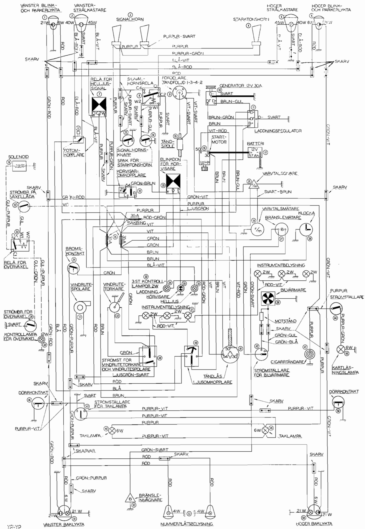
Bildtafel I Elektrischer Schaltplan ab Fahrgestell-Nr. 1 bis Fahrgestell-Nr. 7000
