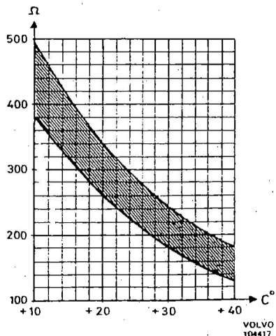
Widerstand im Temperaturfühler für Ansaugluft
