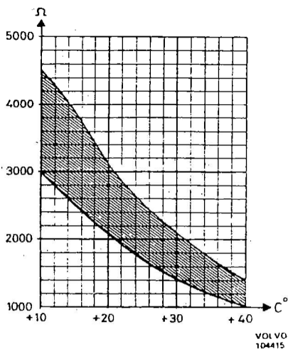
Widerstand im Temperaturfühler für Kühflüssigkeit
