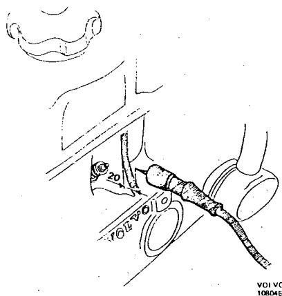
Prüfung der Zündspannung ohne Instrument
