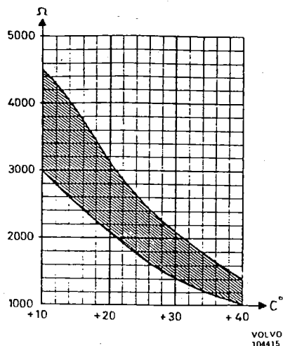
Widerstand im Temperaturfühler für Kühlflüssigkeit
