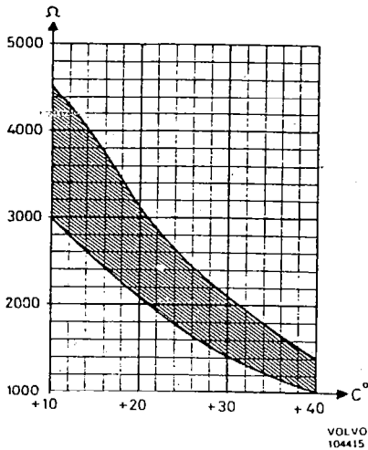
Widerstand im Temperatursensor für Kühflüssigkeit
