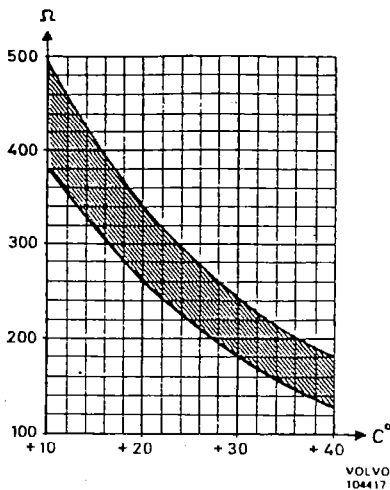
Widerstand im Temperaturfühler für Ansaugluft
