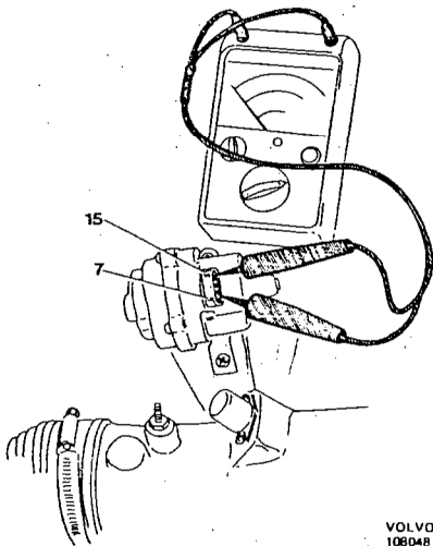
Prüfung des Druckfühlers Der Widerstand in der Primärwicklung soll ca. 90 Ohm betragen.
