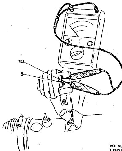
Prüfung des Druckfühlers Der Widerstand in der Sekundärwicklung soll ca. 350 Ohm betragen.
