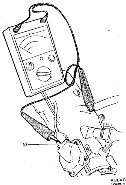
Prüfung des Drosselklappenschalters
