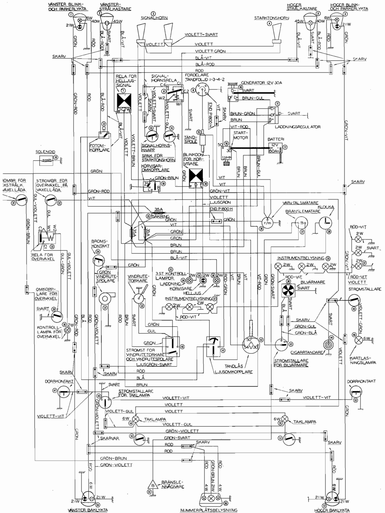
Bildtafel III Elektrischer Schaltplan ab Fahrgestell-Nr. 10001 bis Fahrgestell-Nr. 12500
