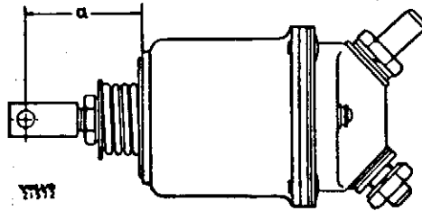
Einstellung des Magnetschalters (Weicheisenkern eingezogen)
