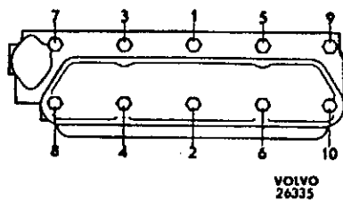
Anziehfolge für Zylinderkopfschrauben, Motor B 18
